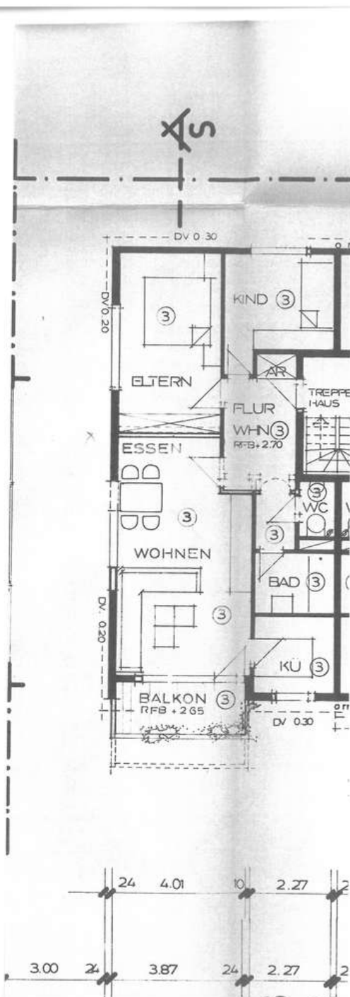
Grundriss
